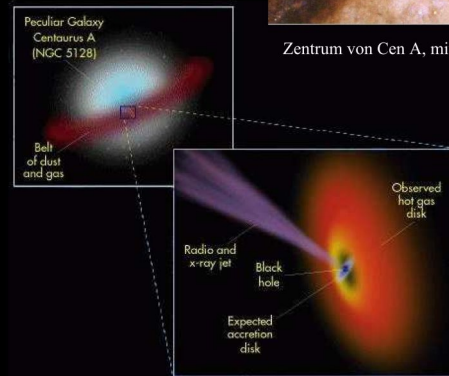
Rekonstruktion: das Schwarze Loch in Cen A mit Jet
